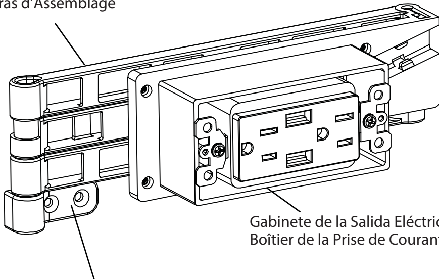
Soporte Desmontable del Gabinete Trasero (abierto a 95 grados para separarlo) Support de Dos d'Armoire Amovible (ouvrir à 95° pour le retirer)
